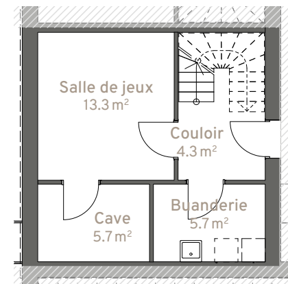
Sous-sol
