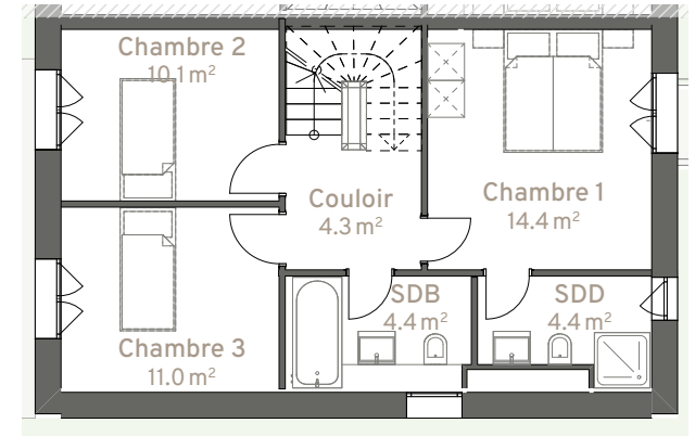
1 er étage
