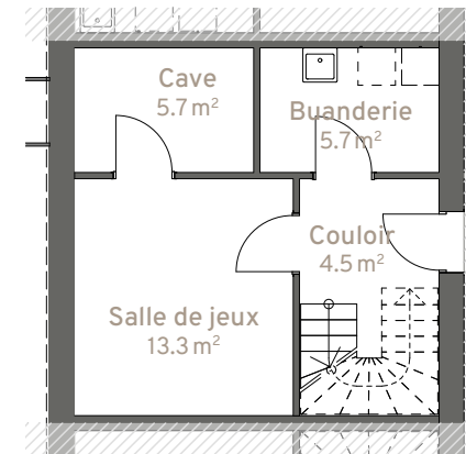
Sous-sol
