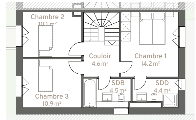
1 er étage
