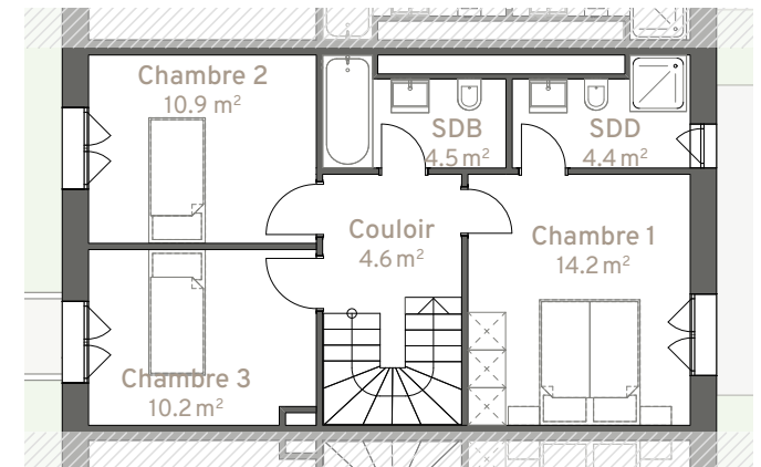
1 er étage
